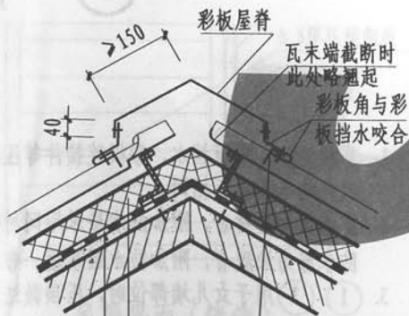
③ 正脊
