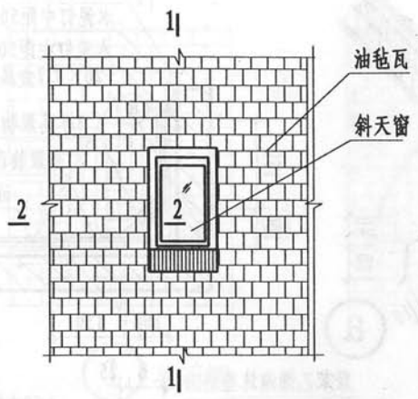
① 平面图
