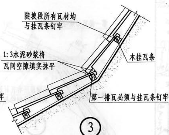
块瓦屋面（木挂瓦条）
