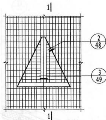
① 平面图
