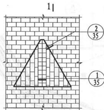
1 平面图
