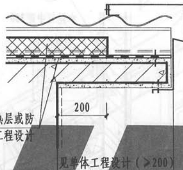
② 山墙挑檐
