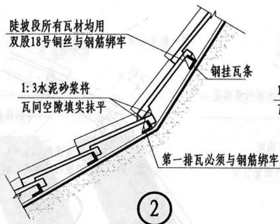
块瓦屋面（钢挂瓦条）
