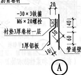
油毡瓦屋面管道泛水(二) 油毡瓦屋面避雷带支架安装
