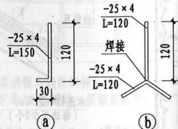
避雷带支架
