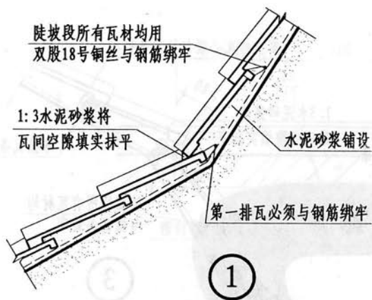
块瓦屋面（砂浆卧瓦）
