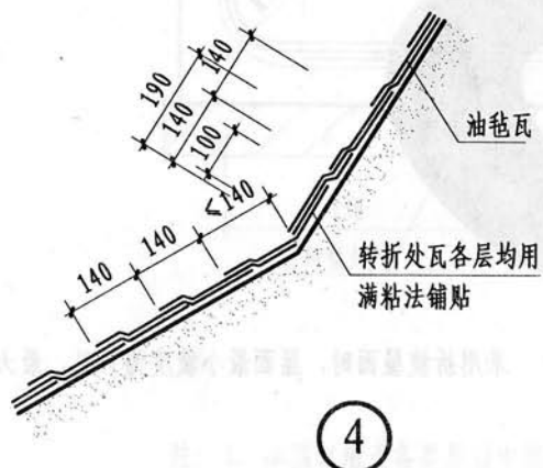
油毡瓦屋面
