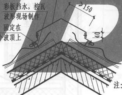
④ 斜脊
