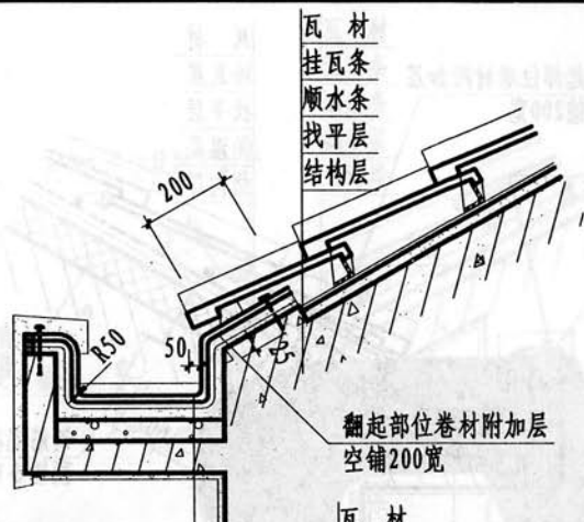
① (无保温层, 无柔性防水层)
