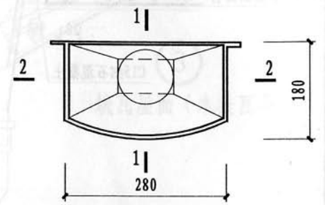
圆(矩)形管雨水斗平面
